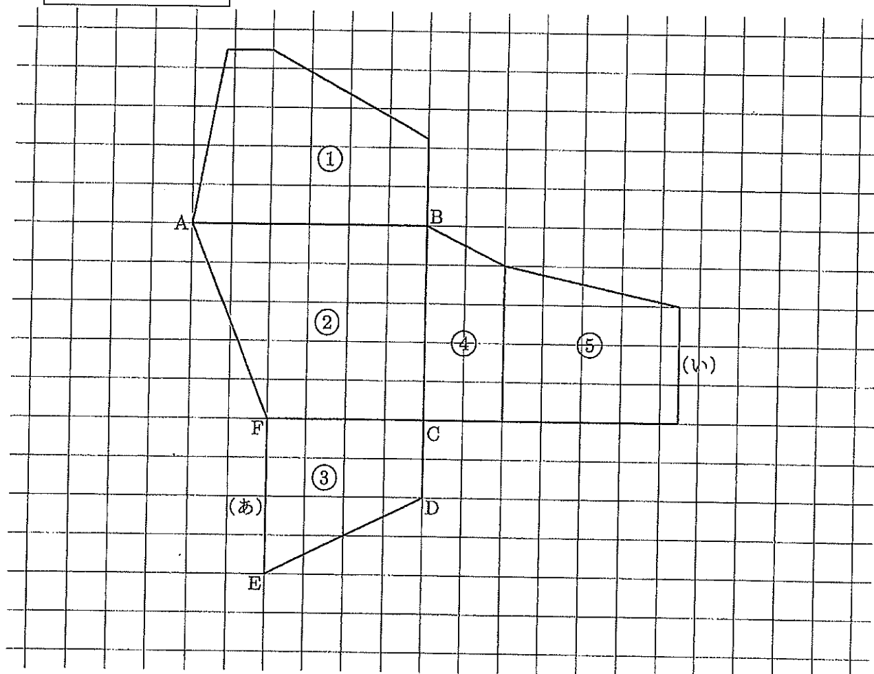
立体 Y の展開図
