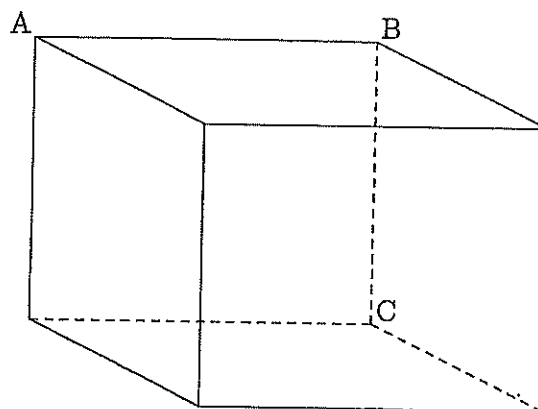
直方体 X の見取図
